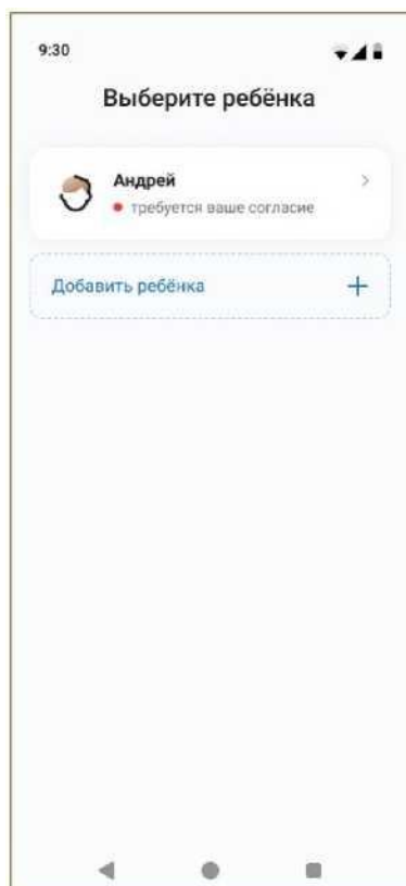
Рисунок 1 - Выбор ребенка
