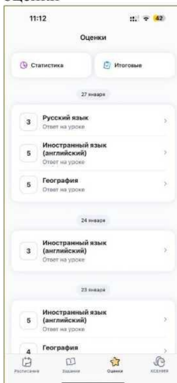
Рисунок 13 - Текущие оценки
